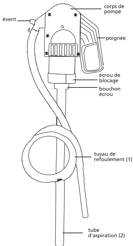
Figure 2 – Illustration de pièces détachées pour Pompe A Levier- Plastique
