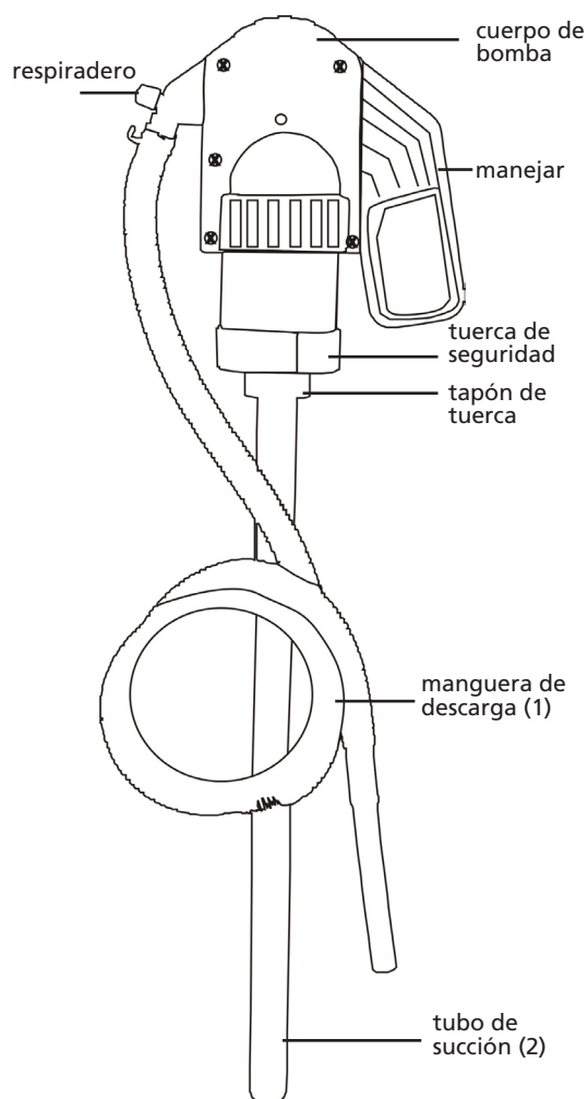
Dibujo 2 – Ilustración de piezas remontas de Bomba Para Transvase -Plastico
