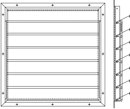
Figure 1 CIRCULATION D'AIR
