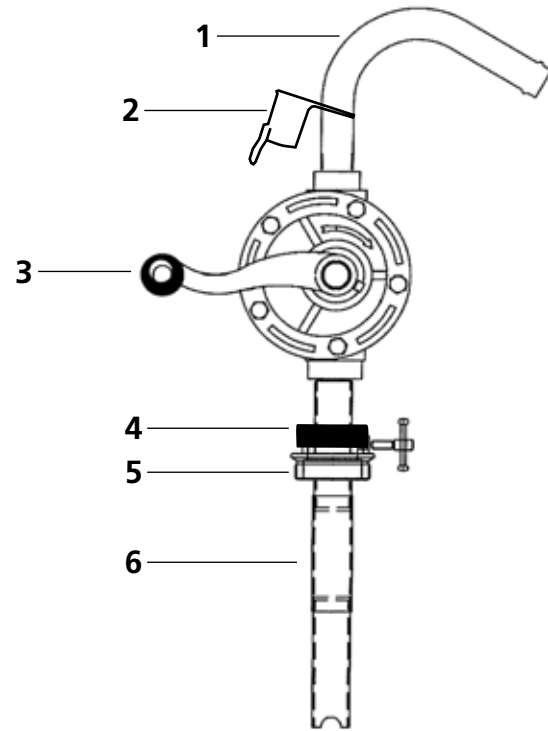
Dibujo 2 - Reparación de piezas de ilustración para Dayton Bomba de Barril Rotativo
