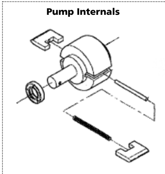
Dibujo 2 - Reparación de piezas de ilustración para Dayton Bomba de Barril Rotativo
