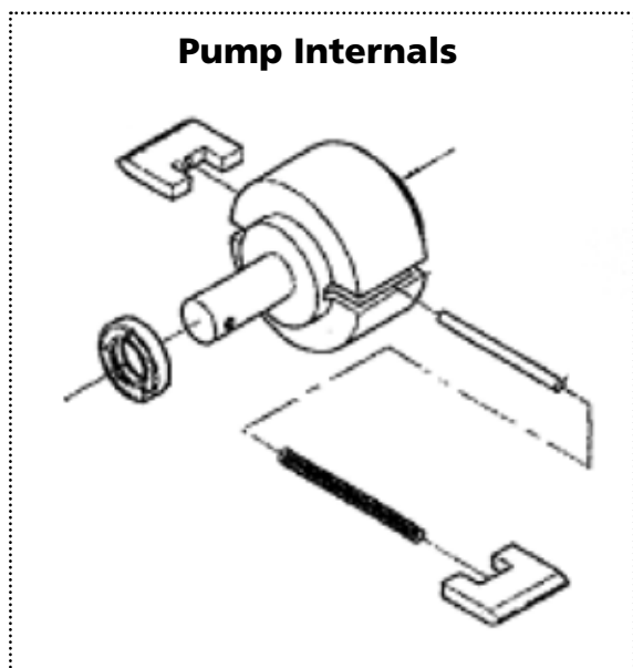
Figure 2 - Illustration des pièces de réparation pour Dayton de pompe Barrel Rotary ®
