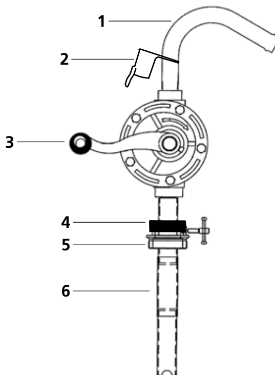
Figure 2 - Illustration des pièces de réparation pour Dayton de pompe Barrel Rotary ®
