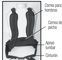
Figura 1 Montaje de la correa
