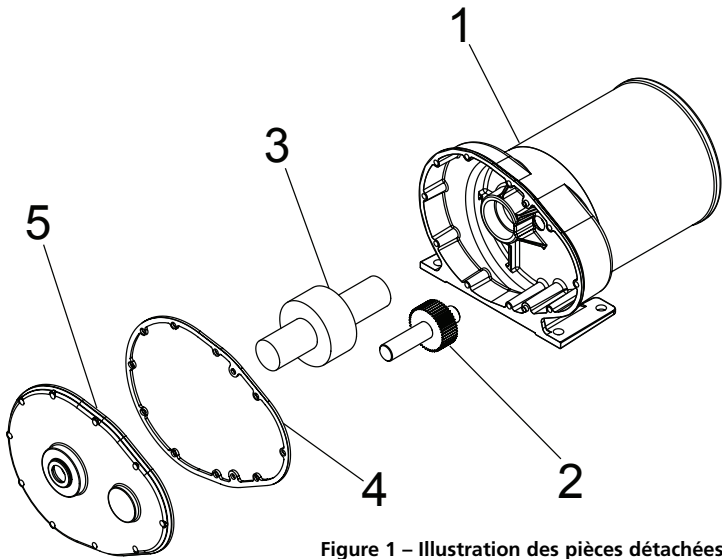
Figure 1 – Illustration des pièces détachées 1LPU3, 1LPU4 et 1LPU5
